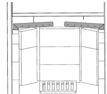
Схема установки трубок дожига «Сибирь-12»
