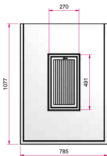
Изображение сверху М 1:20
